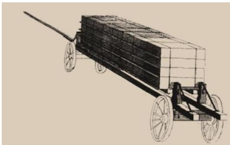
Voz za prevažanje čebelnih panjev (Janša, 1775) – Crane, 1999, str. 350, vir 36
