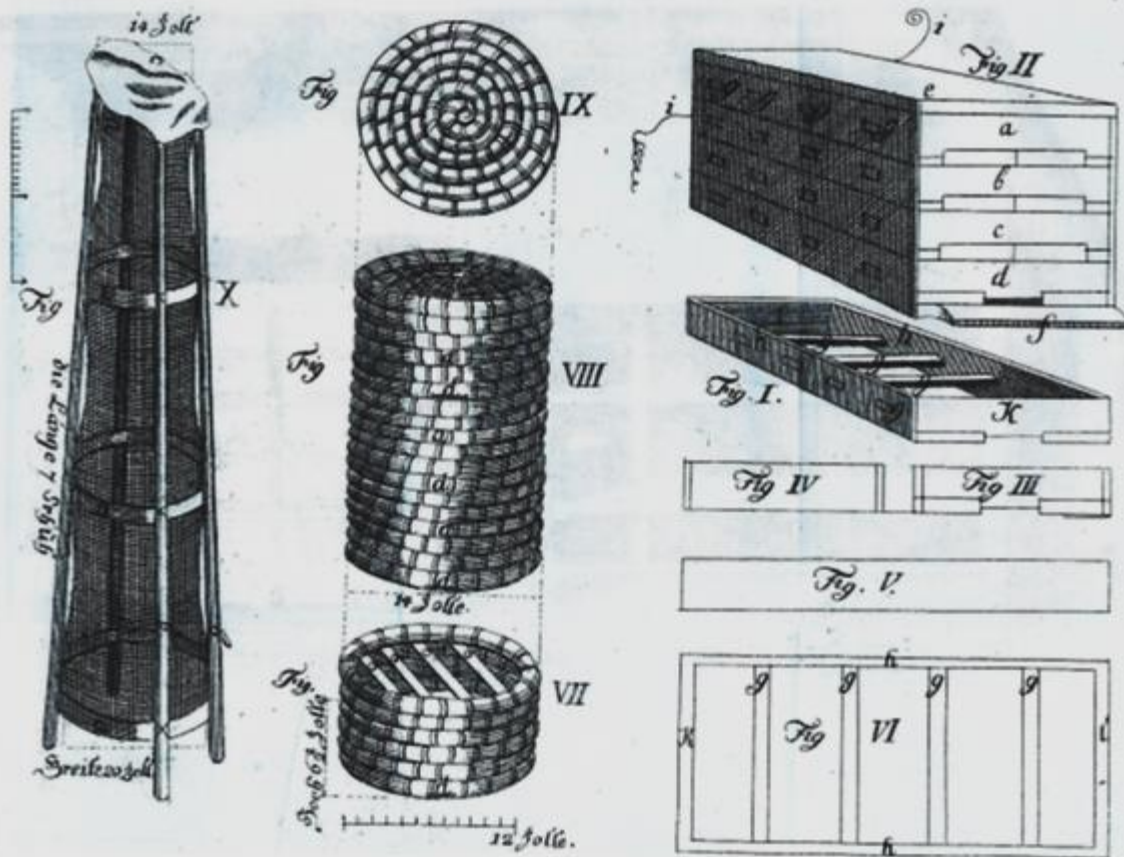
Fig. 1 - polovični panj (obod) s prečnicami (g) Fig. 2 - panj sestavljen iz štirih obodov (a, b, c, d) z žico (i) za prerez satja, pokrit z desko (e) in z dnom (f) Fig. 3 - prednja panjska končnica z izrezanim žrelom Fig. 4 - zadnja panjska končnica Fig. 5 - panjska stranica Fig. 6 - obod s prečnicami (g) Fig. 7 - spodnji slamnati obod z žrelom in štirimi prečnicami Fig. 8 - srednji slamnati obodi (a, d) Fig. 9 - slamnati pokrov Fig. 10 - lovilnik rojev (prestrazalo za roje)
